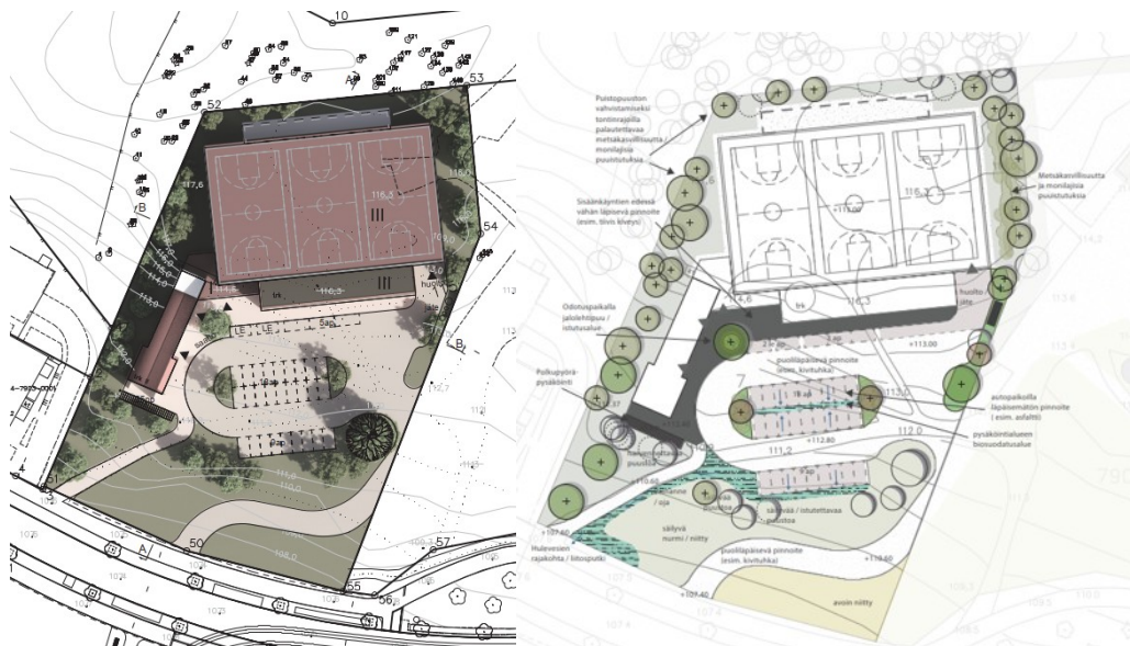
Kuva 3 Liikuntahallin asemapiirros, ehdotusvaihe (vasemmalla) ja sitä vastaava pihasuunnitelma (oikealla). Kuvat: asemapiirros Arkkitehdit Kontukoski Oy ja pihasuunnitelma Tampereen kaupunki.
