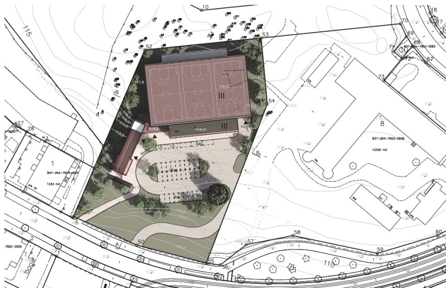
Kuva 14 Asemapiirustus, jossa esitetään liikuntahallin, yhteyksien ja pysäköinnin sijoittuminen tontille. Kuva: Arkkitehdit Kontukoski Oy.
